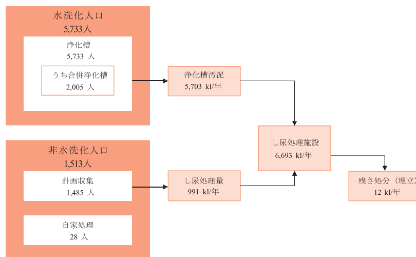
図：し尿処理量(令和元(2019)年度現在)[出典：甘楽西部環境衛生施設組合資料]
