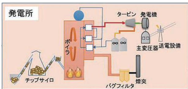
木質バイオマス発電設備の概要
