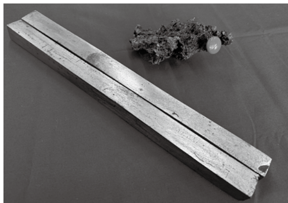
たたらで作ったケラ(右上)と鉄柱
