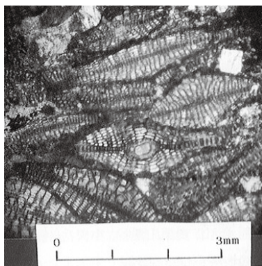
←有孔虫化石の 顕微鏡写真
