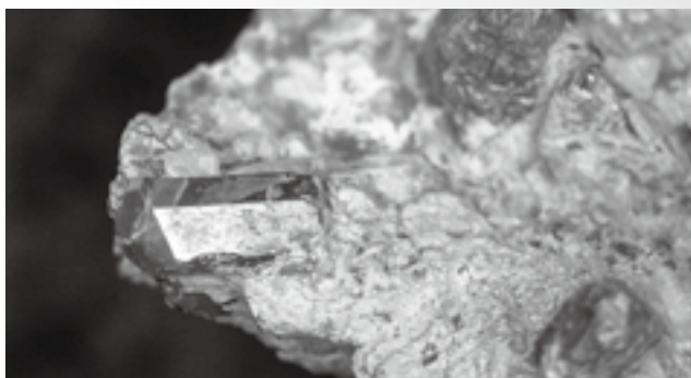
▲西牧鉾山の鶏冠石 （群馬県立自然史博物館所蔵）
